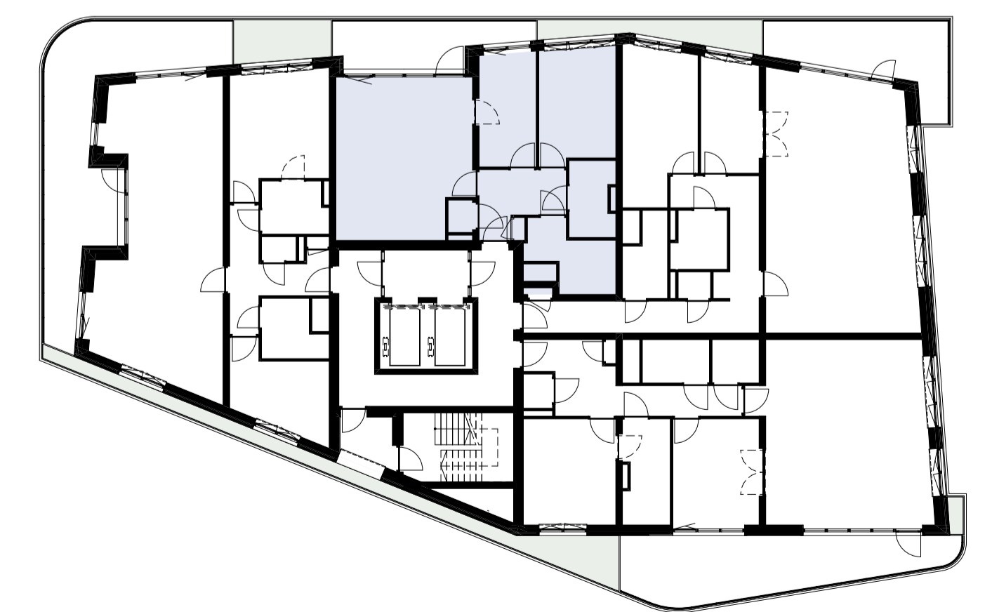
EERSTE VERDIEPING
