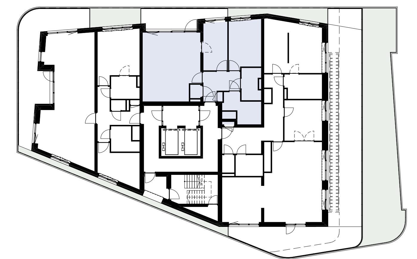
VIJFDE VERDIEPING
