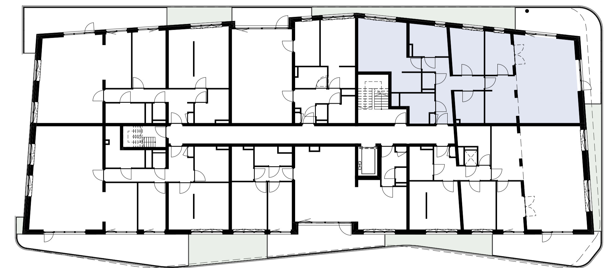
EERSTE VERDIEPING
