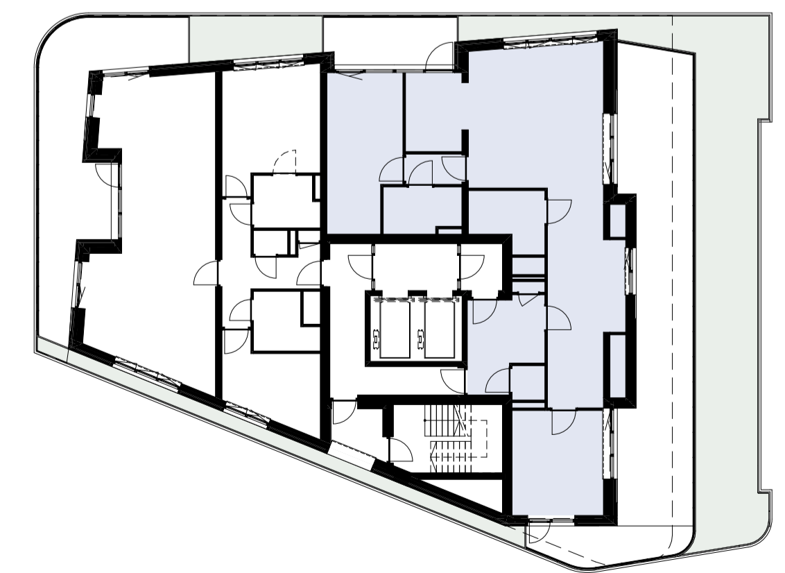
ACHTSTE VERDIEPING
