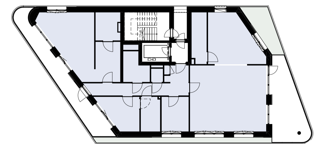
EERSTE VERDIEPING
